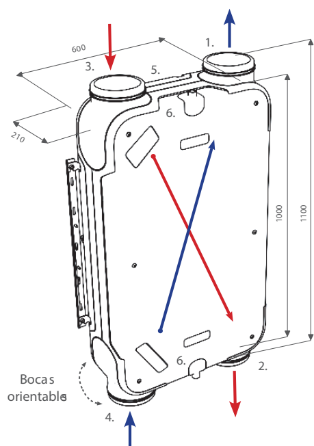
Flujos de aire versión izquierda (versión de fábrica)
